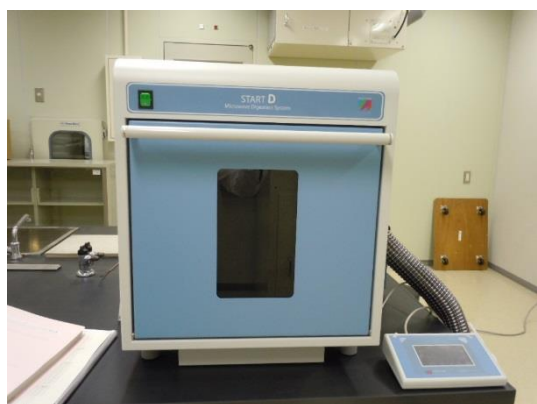
マイクロ波分解前処理装置 スタートD
