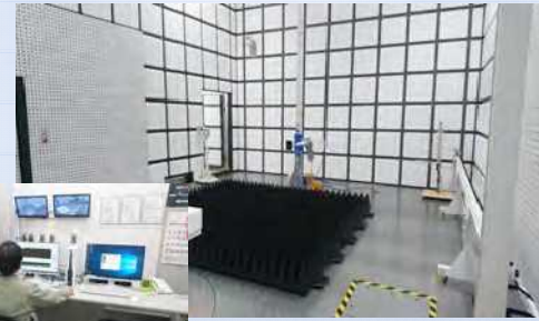
電波暗室
